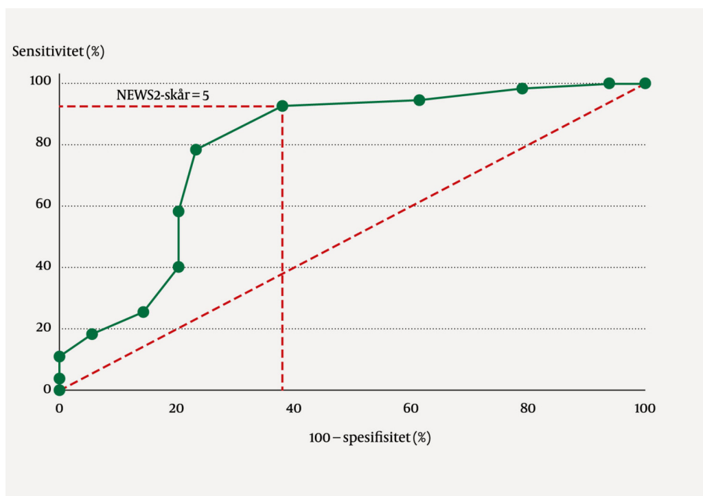
Figur 2 ROC-kurve ( receiver operating characteristic ) som viser hvor god total NEWS2-skår er til å skille pasienter med og uten sepsis. NEWS2-skår på 5, som er anbefalt varslingsterskel,
